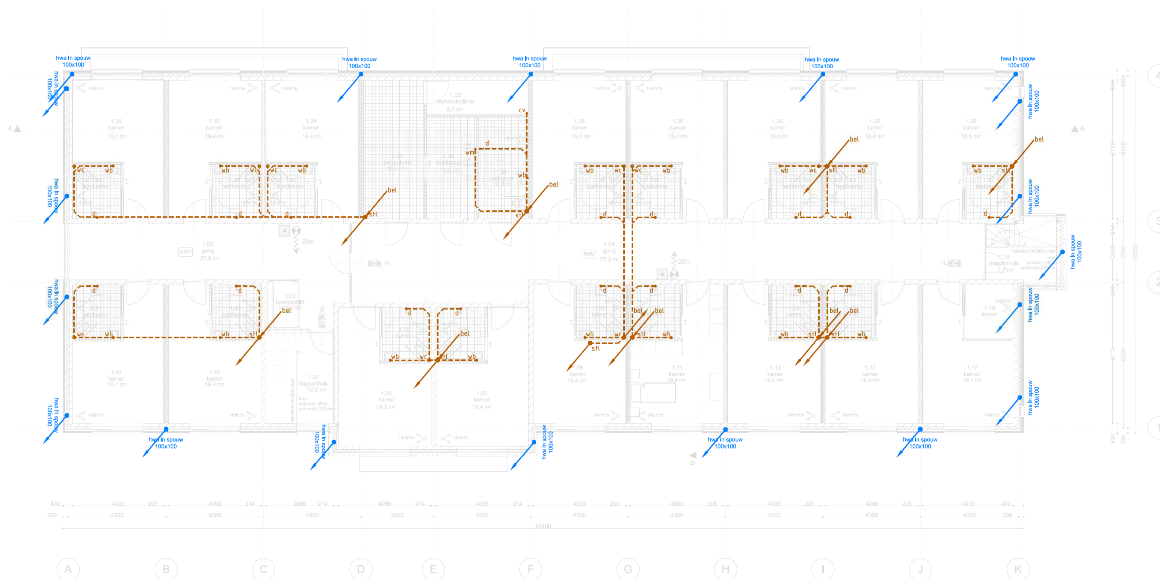
eerste verdieping 3030+ peil BVO = 884 m²
