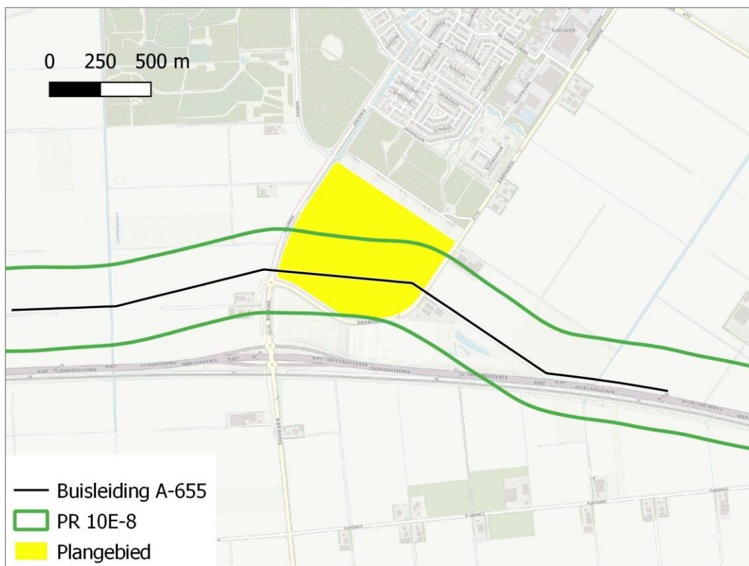
Figuur 3. PR-contouren aardgasleiding W-655
