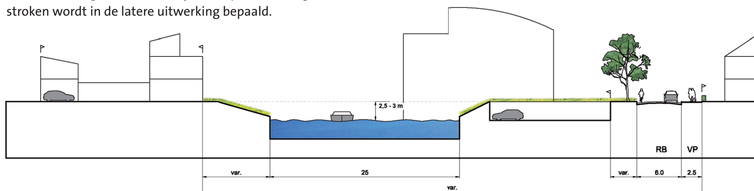
Doorsnede DD': waterwonen aan de insteekhaven
